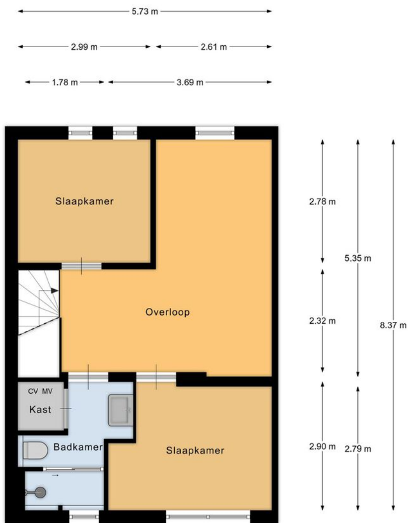
2e verdieping
