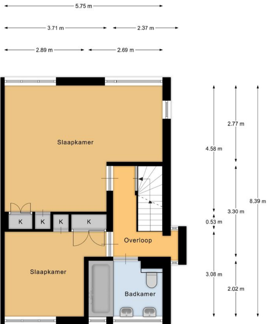
1e verdieping
