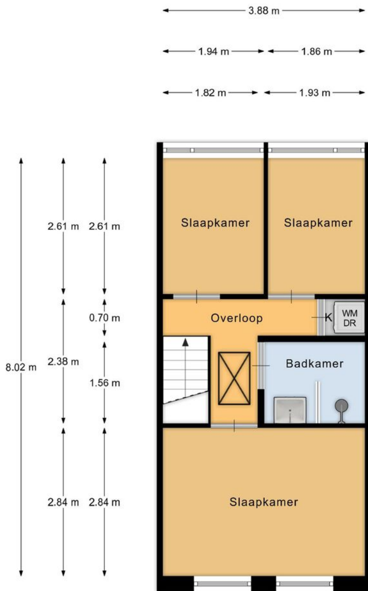
1e verdieping
