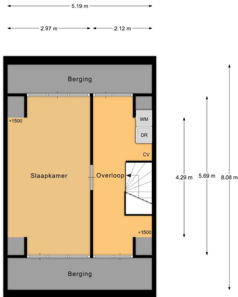
2e verdieping
