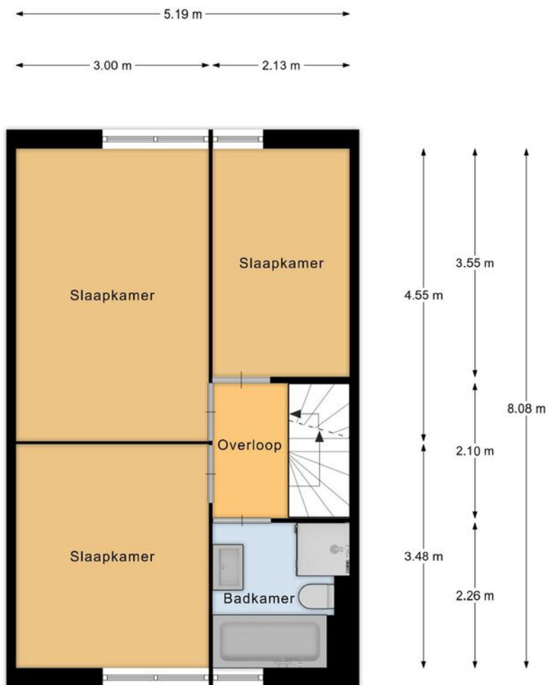
1e verdieping
